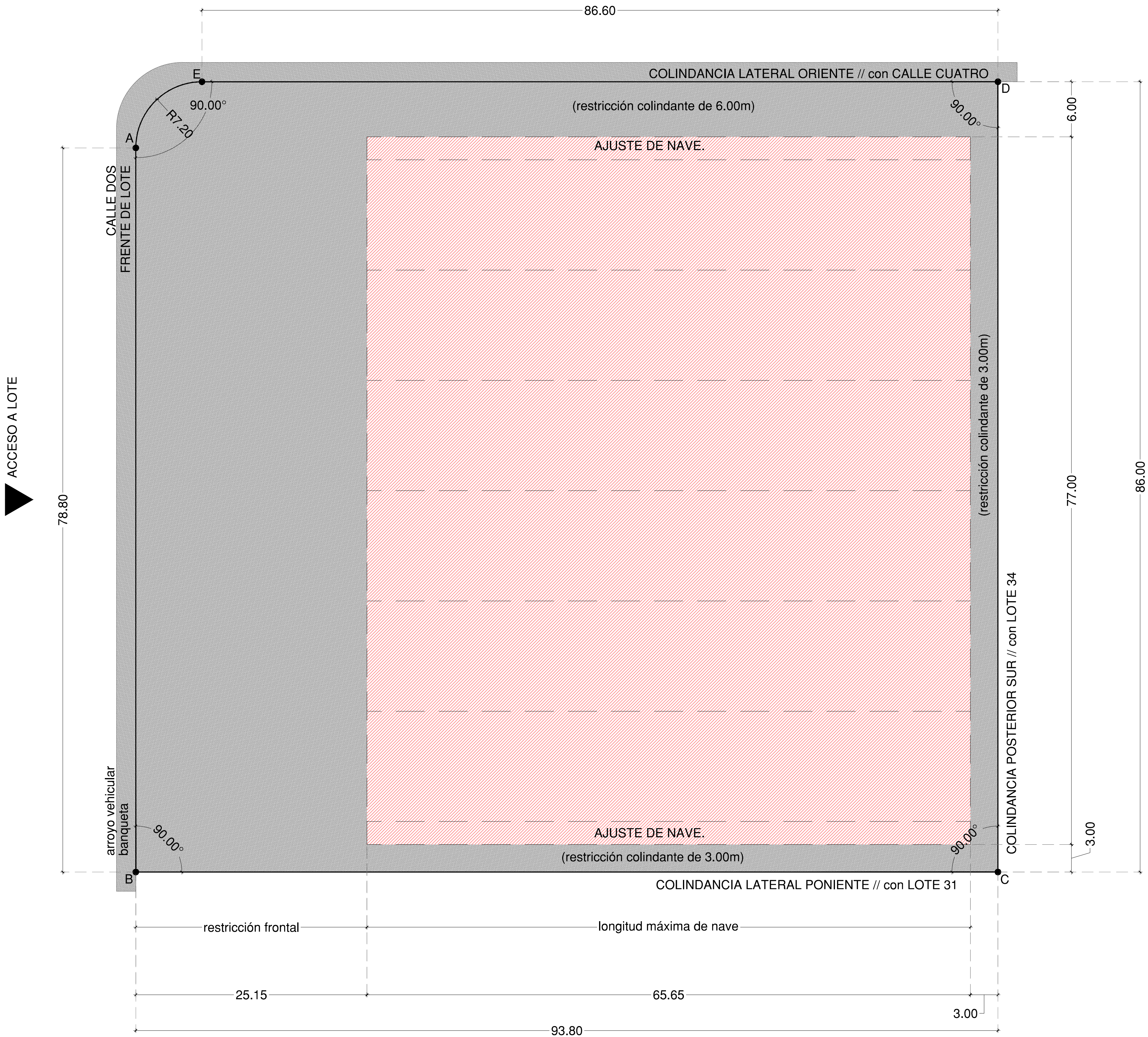
PLANTA > LOTE 33 ESCALA 1:250 PIA // PARQUE INDUSTRIAL AEROPUERTO, QRO.-MX
